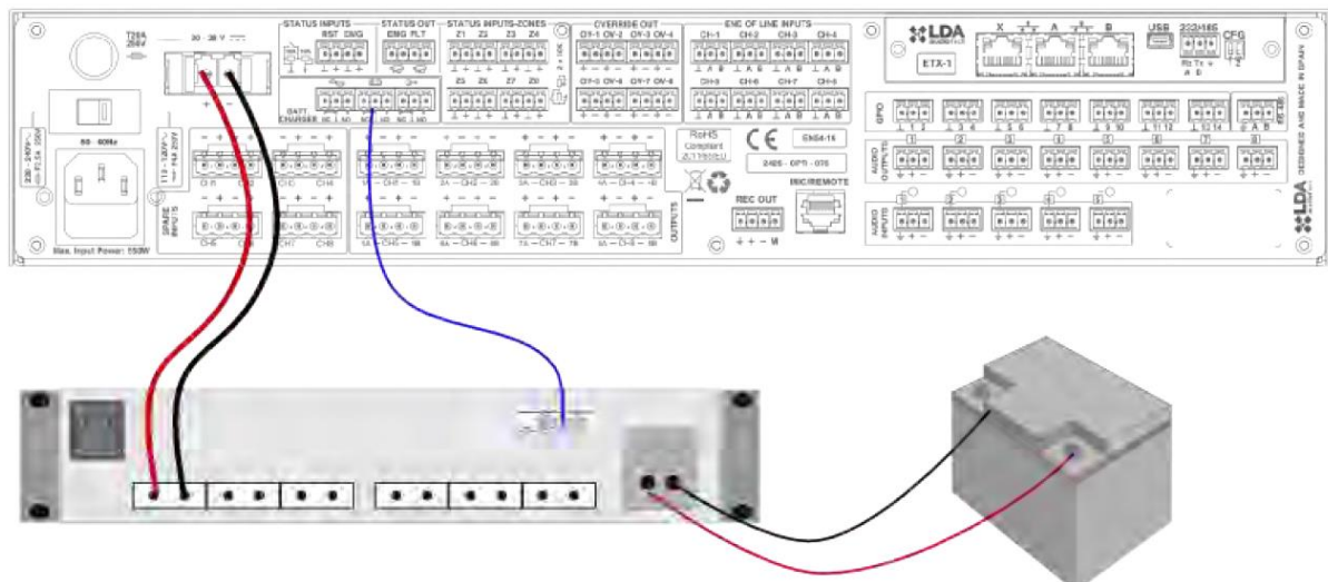
Abbildung 41 Prinzipbild Notstromversorgung
