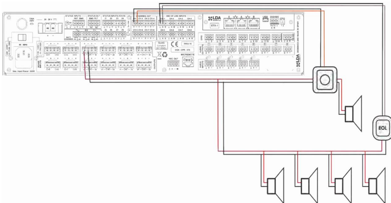
Abbildung 50 Prinzipbild Anschluss mehrerer EoL-Modul an eine Lautsprecherlinie
