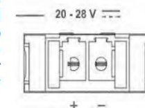
Abbildung 21: DC-Notstrom-Einspeisung
