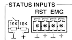
Abbildung 10: Notfall -Schnittstelle
