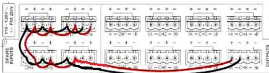
Abbildung 44 Prinzipbild HAVARIEVERSTÄRKER
