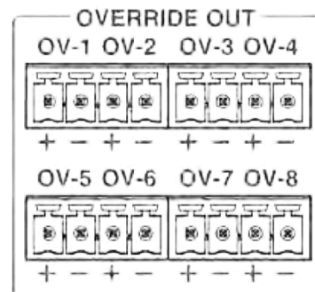
Abbildung 13: Override-Ausgänge
