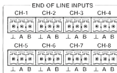
Abbildung 14: EOL-Inputs
