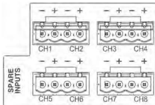
Abbildung 22: Havarieverstärker-Eingang
