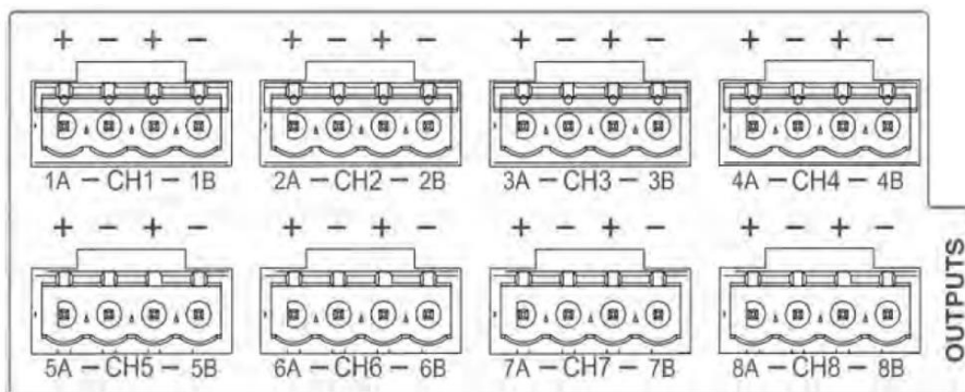
Abbildung 23: Ausgänge der Lautsprecherlinien
