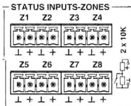
Abbildung 12: Notfall-Schnittstelle Z1-Z8
